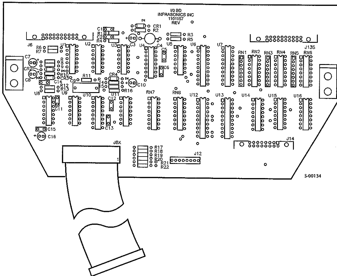
Figure 7-13. I/O (Input/Output) PCA
